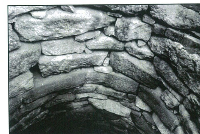
挖到含水層，避免井倒塌，在邊緣 用石頭或磚頭堆疊
